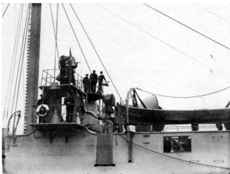
Фрагмент правого борта крейсера «Диана»: кормовая прожекторная площадка и порт 75-мм палубного орудия, примерно 1908 г.
