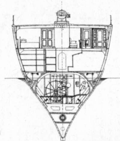
ПОПЕРЕЧНОЕ СЪЧЕНИЕ № 119.
