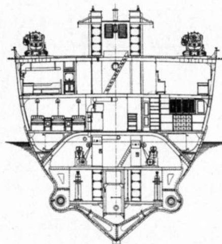
ПОПЕРЕЧНОЕ СЪЧЕНИЕ № 109.
