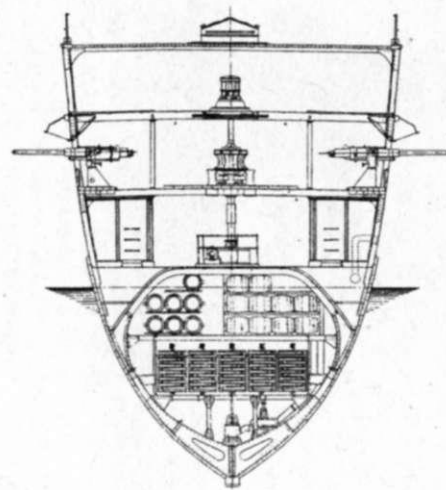
ПОПЕРЕЧНОЕ СЪЧЕНИЕ № 96.
