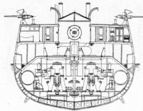
ПОПЕРЕЧНОЕ СЪЧЕНИЕ № 79.
