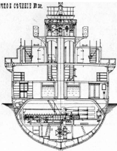
Поперечные сечения крейсера 1 ранга «Диана» Копии подлинных чертежей
