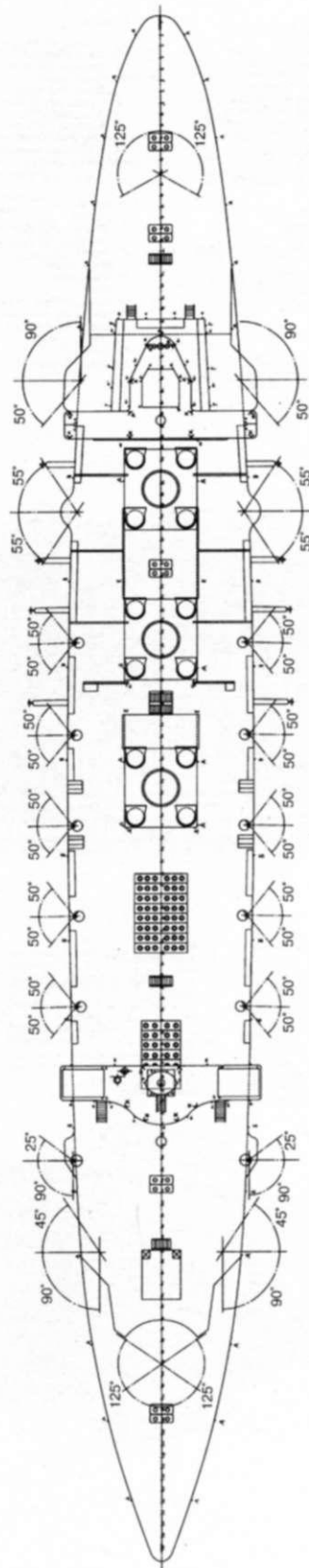
Крейсер 1 ранга «Диана» Боковой вид и вид сверху с указанием секторов обстрела
