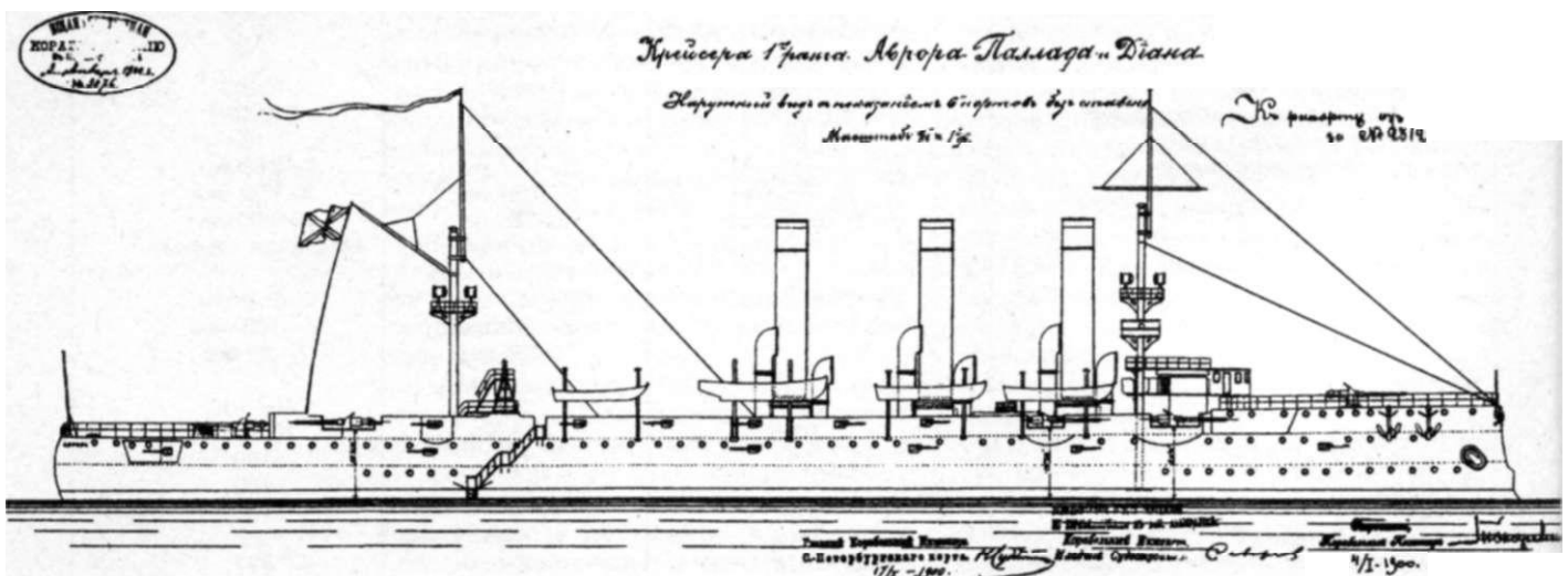
Крейсер типа «Диана»: боковой вид и план носового мостика по первоначальному проекту, 1899 г.
