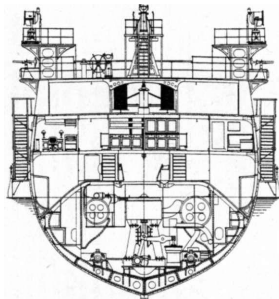
ПОПЕРЕЧНОЕ СЪЧЕНИЕ № 96.
